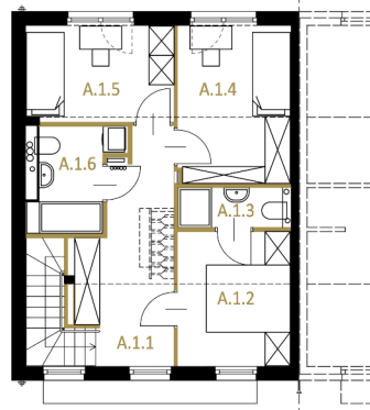
RZUT PODDASZA
