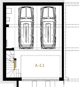
RZUT PIWNICY
