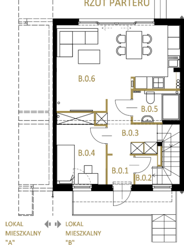
RZUT PARTERU
