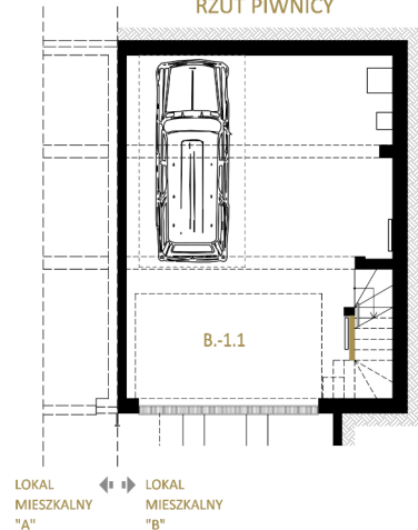
RZUT PIWNICY
