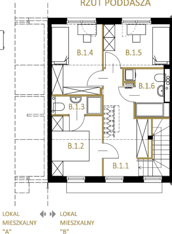
RZUT PODDASZA
