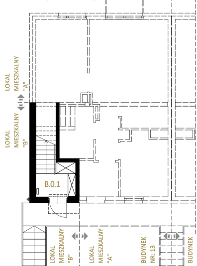
RZUT PARTERU
