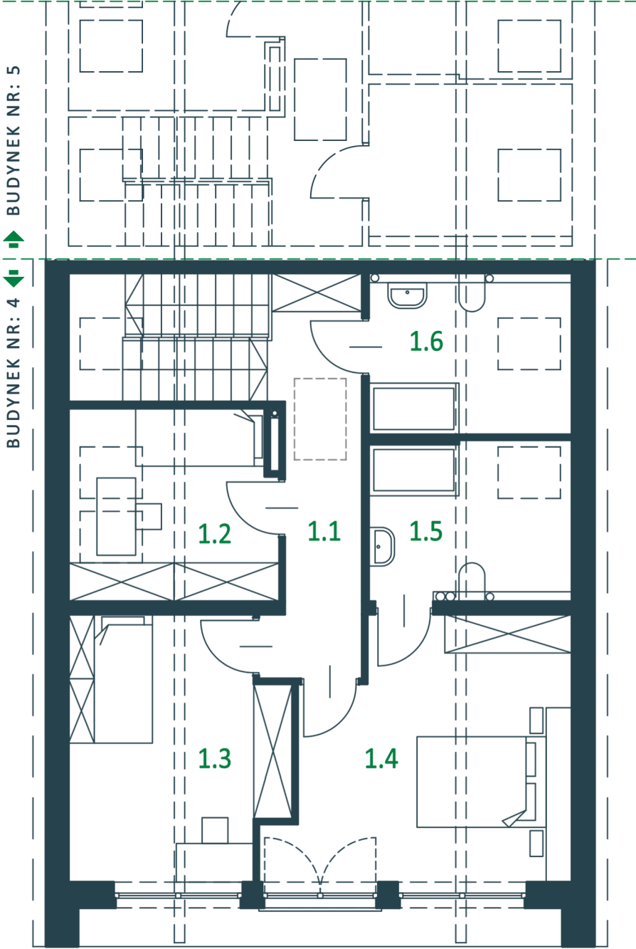
RZUT PODDASZA
