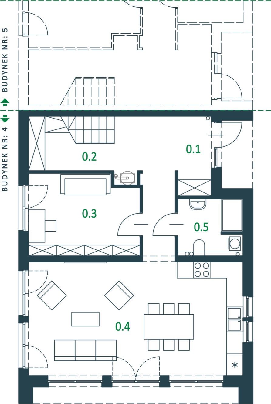
RZUT PARTERU
