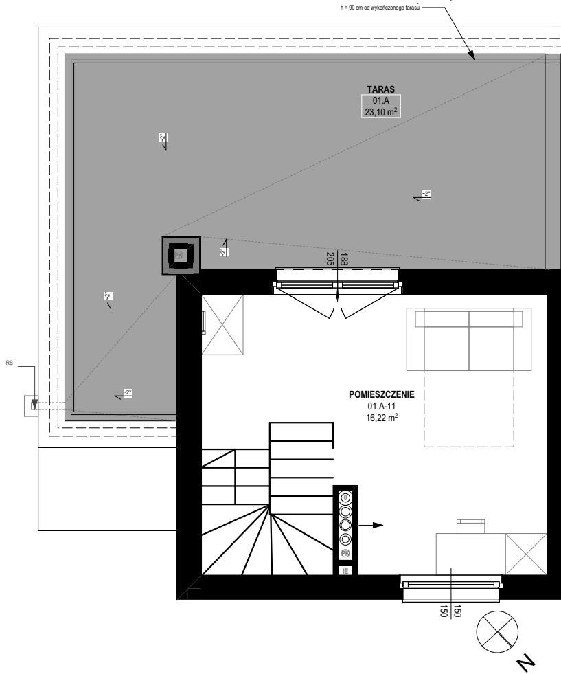
RZUT 2 PIĘTRA
