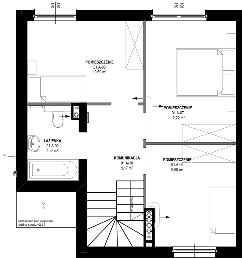
RZUT 1 PIĘTRA
